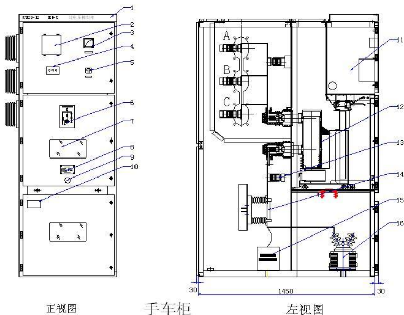
1、眉头 2、智能微机装置 3、电压表 4、高压带电显示器 5、电压转换开关 6、一次模拟牌 7、观察窗 8、铜铭牌 9、断路器手车摇把孔 10、柜内照明灯 11、仪表室 12、隔离手车 13、电压传感器 14、PT快速熔断器 15、大容量综合过电压保护器 16、电压互感器
