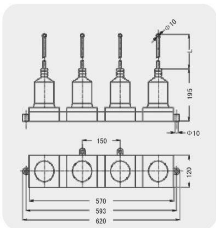
图3 6kV、10kV组合式过电压保护器外形图(T型)
