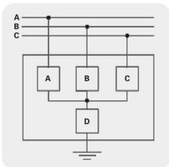
图1 组合式过电压保护器原理图
