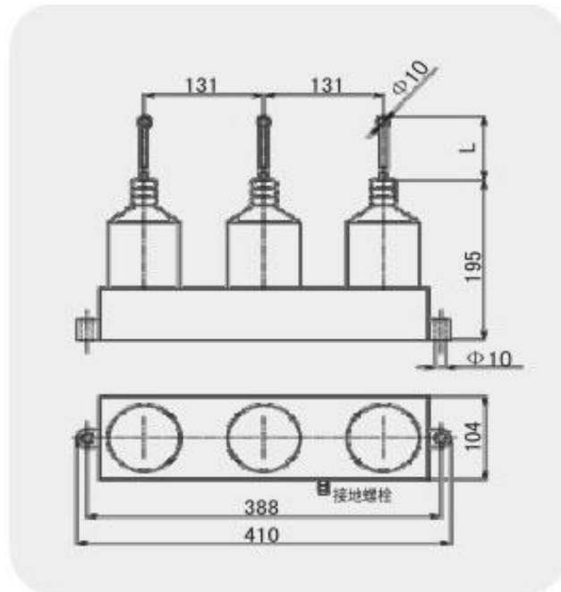
图7 6kV、10kV组合式过电压保护器外形图(三柱式)
