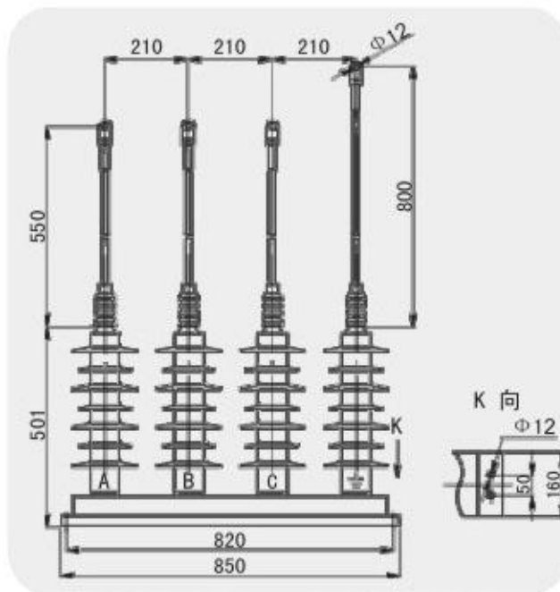
图6 35kV组合式过电压保护器外形图
